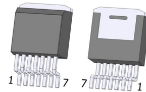
TO-263-7 CASE 418BA
