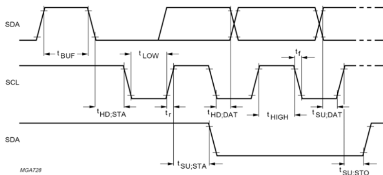
图 18 I 2 C 总线定时波形
