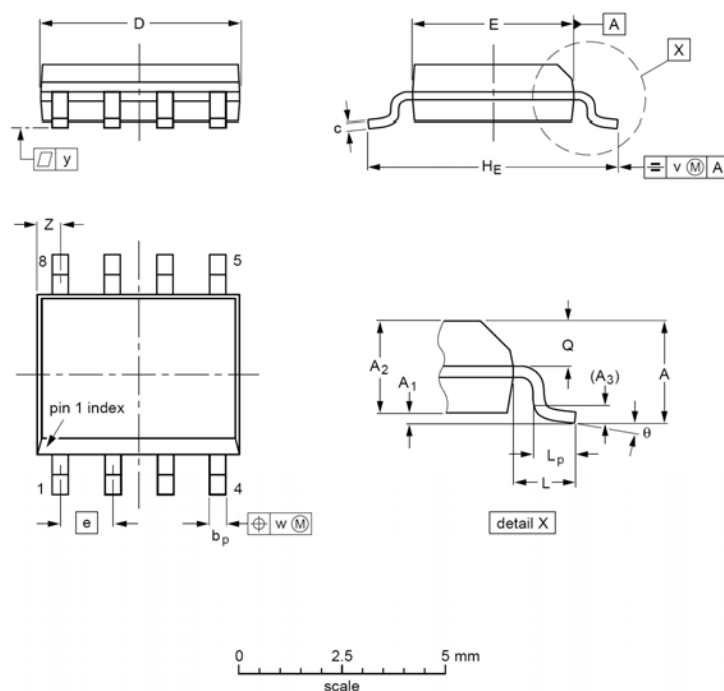
图 19 SOP-8
