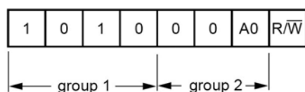
图 10 HTC8563 的器件地址字节的组成
