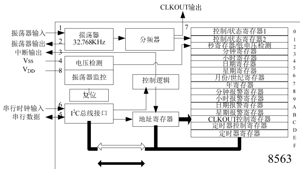
图 1 HTC8563 电路结构框图
