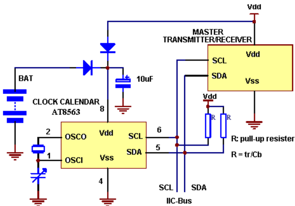
图 为 HTC8563 的应用简图。
