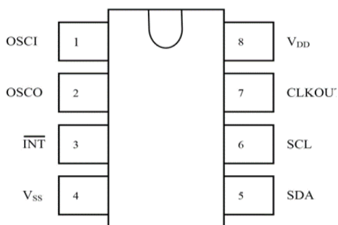
图 2 HTC8563 的引脚排列顺序
