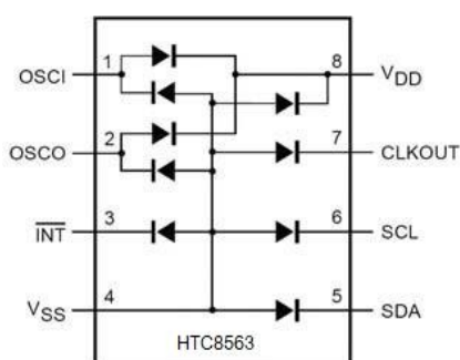
图 3 二极管保护图
