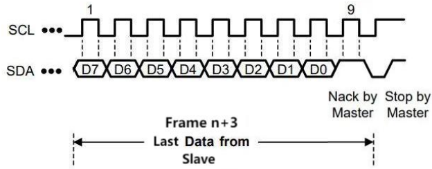
图 7.2-2 I2C 连续读取时序
