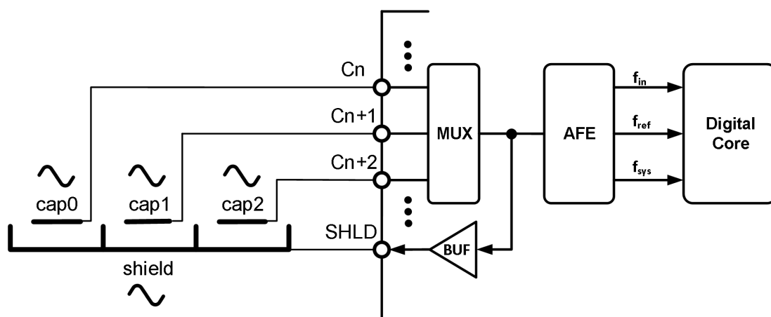
图 6.3.9-2 模式 2-多路有源屏蔽
