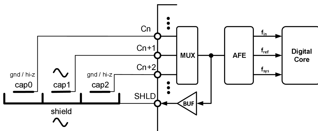
图 6.3.9-1 模式 1-单路有源屏蔽
