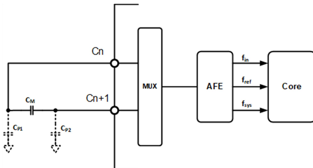
图 6.3.3.3-1 测量互电容
