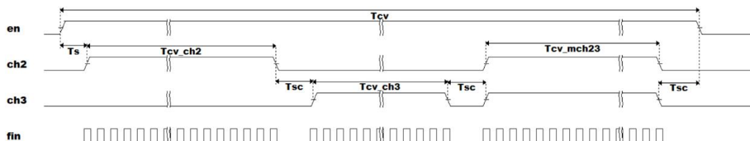
图 6.3.4-2 互电容测量工作流程
