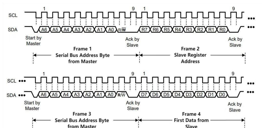
图 7.2-1 I2C 读取时序
