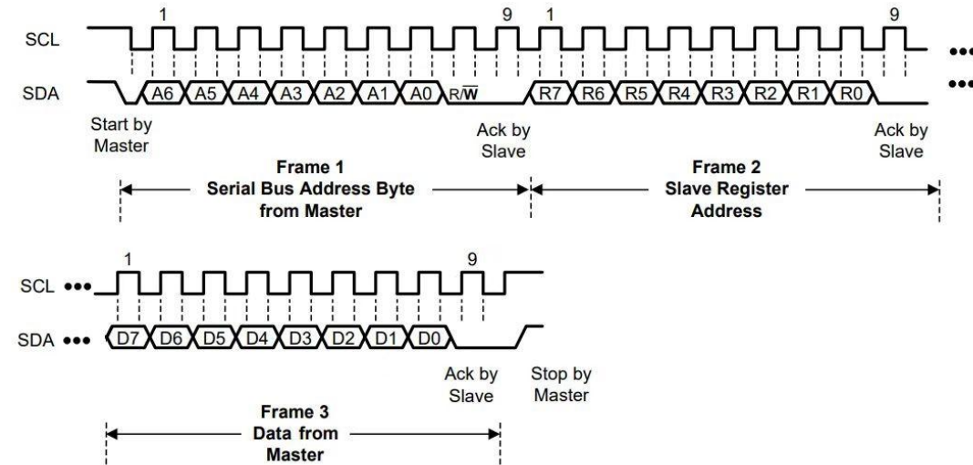
图 7.2-3 I2C 写时序
