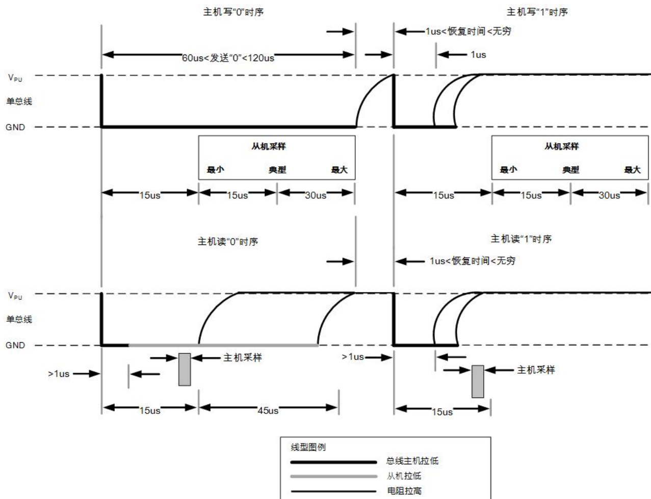
图 11.6-2 读/写时序
