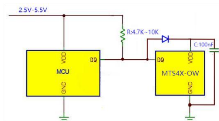
图 9.9 寄生模式典型电路图
