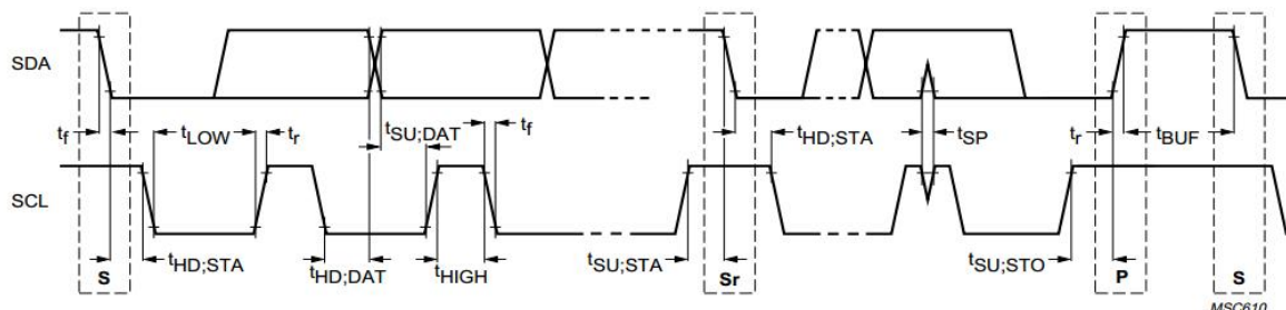
图 11.3 I 2 C 时序参数
