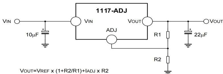
图 2. 典型可调输出电压
