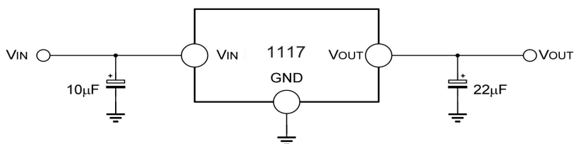
图 1. 典型固定输出电压
