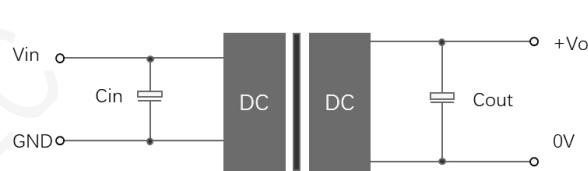
图 4: 应用电路
