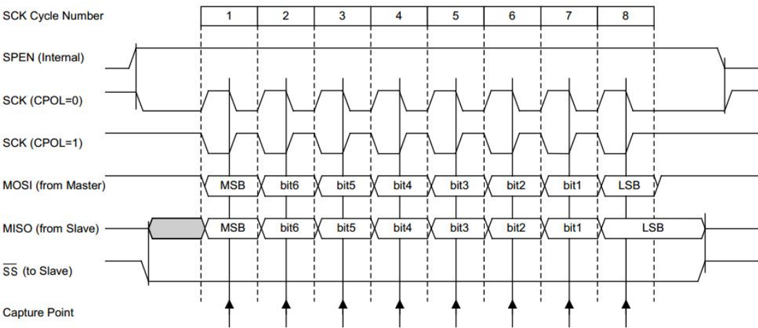
Figure 16-4 数据发送形式（CPHA=1）
