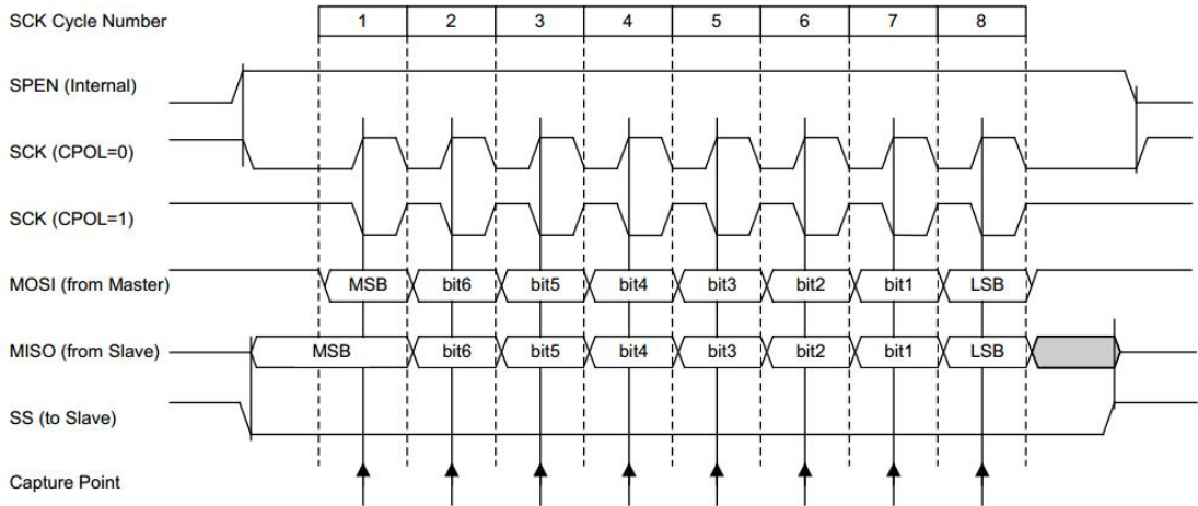
Figure 16-3 数据传送形式（CPHA=0）
