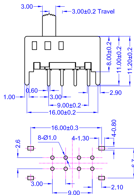
P.C.B LAYOUT
