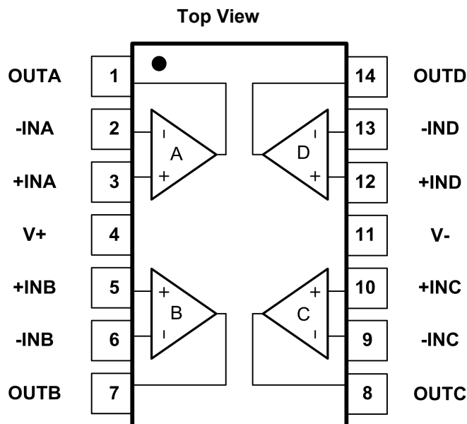
Fig.4-4. GT8534: PD(SOP14) Package GT8534: TD(TSSOP14) Package
