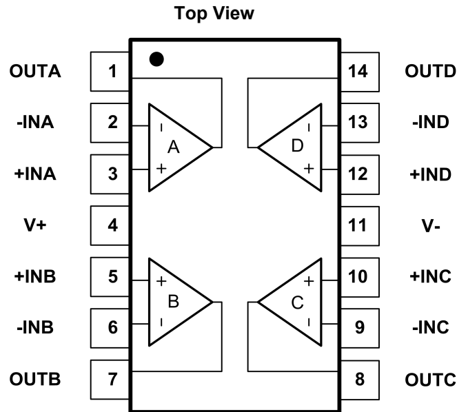
Fig.4-4. GT8564: PD(SOP14) Package GT8564: TD(TSSOP14) Package
