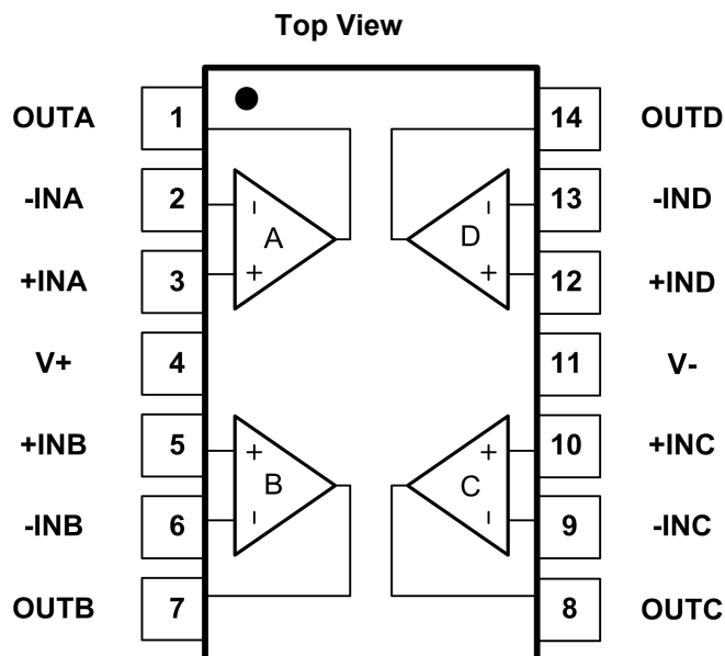
Fig.4-4. GT8554: PD(SOP14) Package GT8554: TD(TSSOP14) Package
