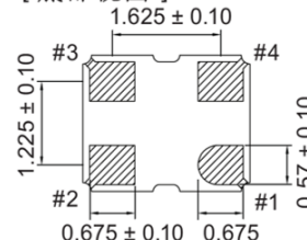
[ 底部视图 ]
