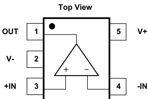
Fig.4-1. GT8501: S5(SOT23-5) Package
