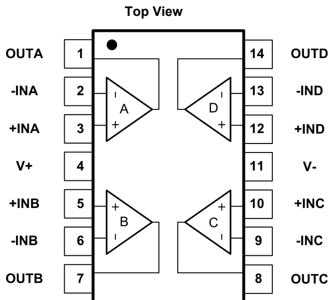
Fig.4-4. GT8504: PD(SOP14) Package GT8504: TD(TSSOP14) Package
