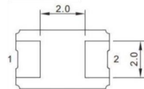
底部视图
