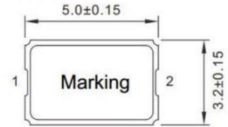
侧视图
