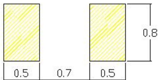
建议焊盘尺寸
