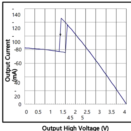
接收器输出电流与输出高电压关系
