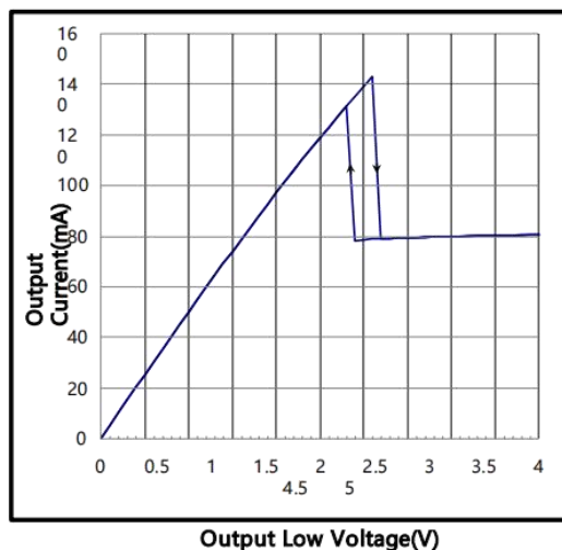
接收器输出电流与输出低电压关系
