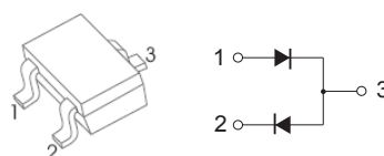
SOT-323
