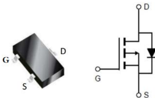
SOT23-3L
