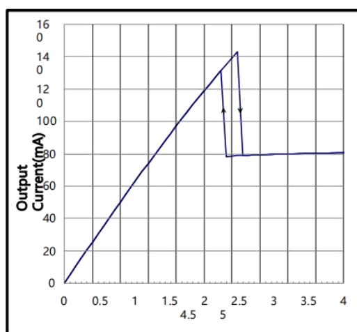
驱动器输出电流与输出低电压关系
