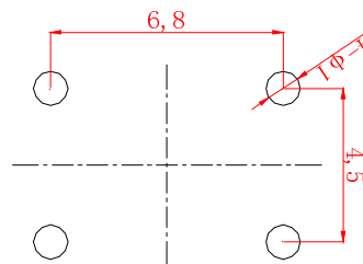
PCB参考图
