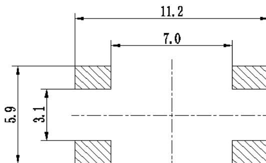
安装尺寸图
