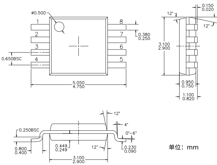
图 15: 封装 MSOP8
