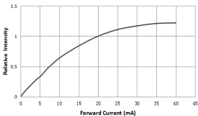
相对光强与电流特性曲线
