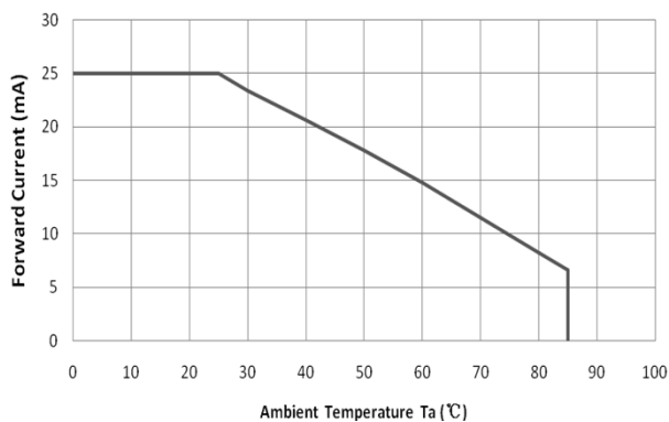
最大正向电流与环境温度特性曲线
