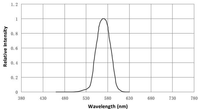
光谱分布特性曲线
