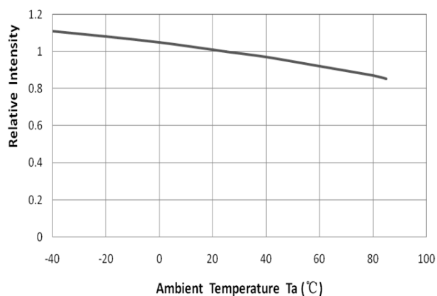
相对光强与环境温度特性曲线
