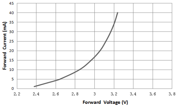
伏安特性曲线
