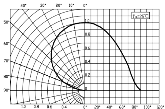
辐射特性曲线
