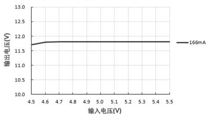
输出电压 VS 输入电压 (IB0512S-2WR3)
