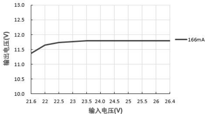
输出电压 VS 输入电压 (IB2412S-2WR3)
