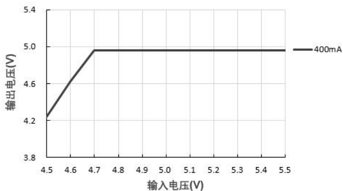
输出电压 VS 输入电压 (IB0505S-2WR3)
