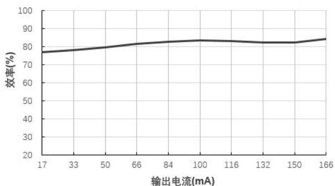
效率 VS 输出电流 IB2412S-2W@ (Vin=24V)
