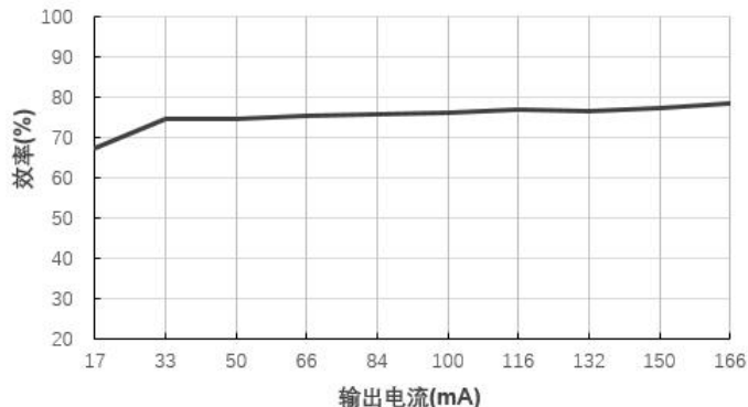
效率 VS 输出电流 IB0512S-2W@ (Vin=5V)
