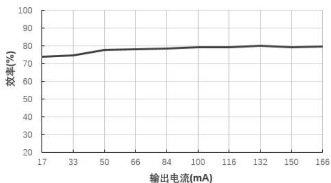
效率 VS 输出电流 IB1212S-2W@ (Vin=12V)
