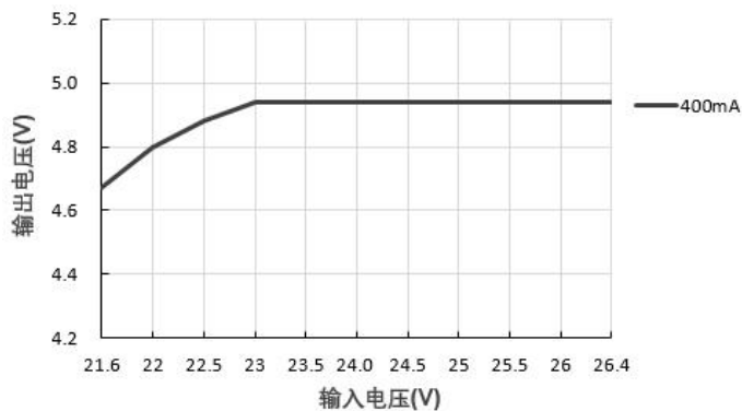
输出电压 VS 输入电压 (IB2405S-2WR3)
