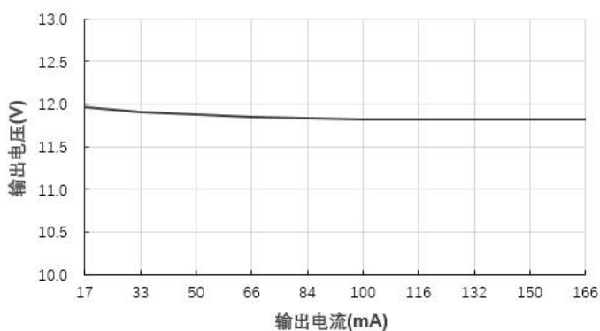
输出电压 VS 输出电流 IB2412S-2W@ (Vin=24V)
