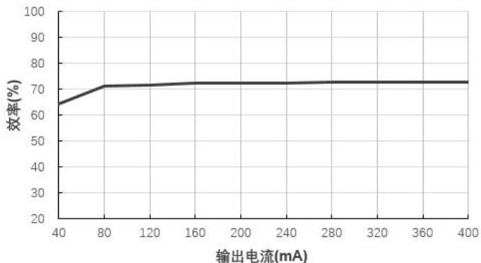
效率 VS 输出电流 IB1205S-2W@ (Vin=12V)
