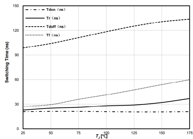
Typ.Switching times vs temperature/开关时间与结温特性
