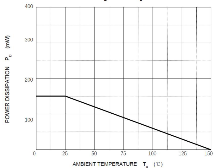
P_D — T_a
