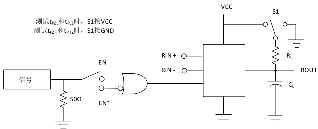
图 3. 三态延时测试电路
