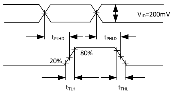
图 2. 传输延时和转变时间波形图
