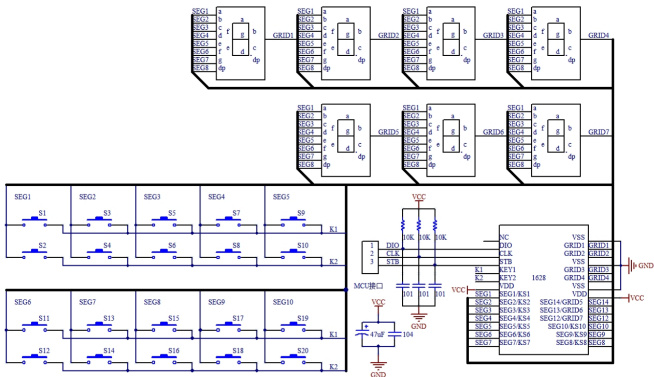
1628驱动共阴数码管接线电路图:
