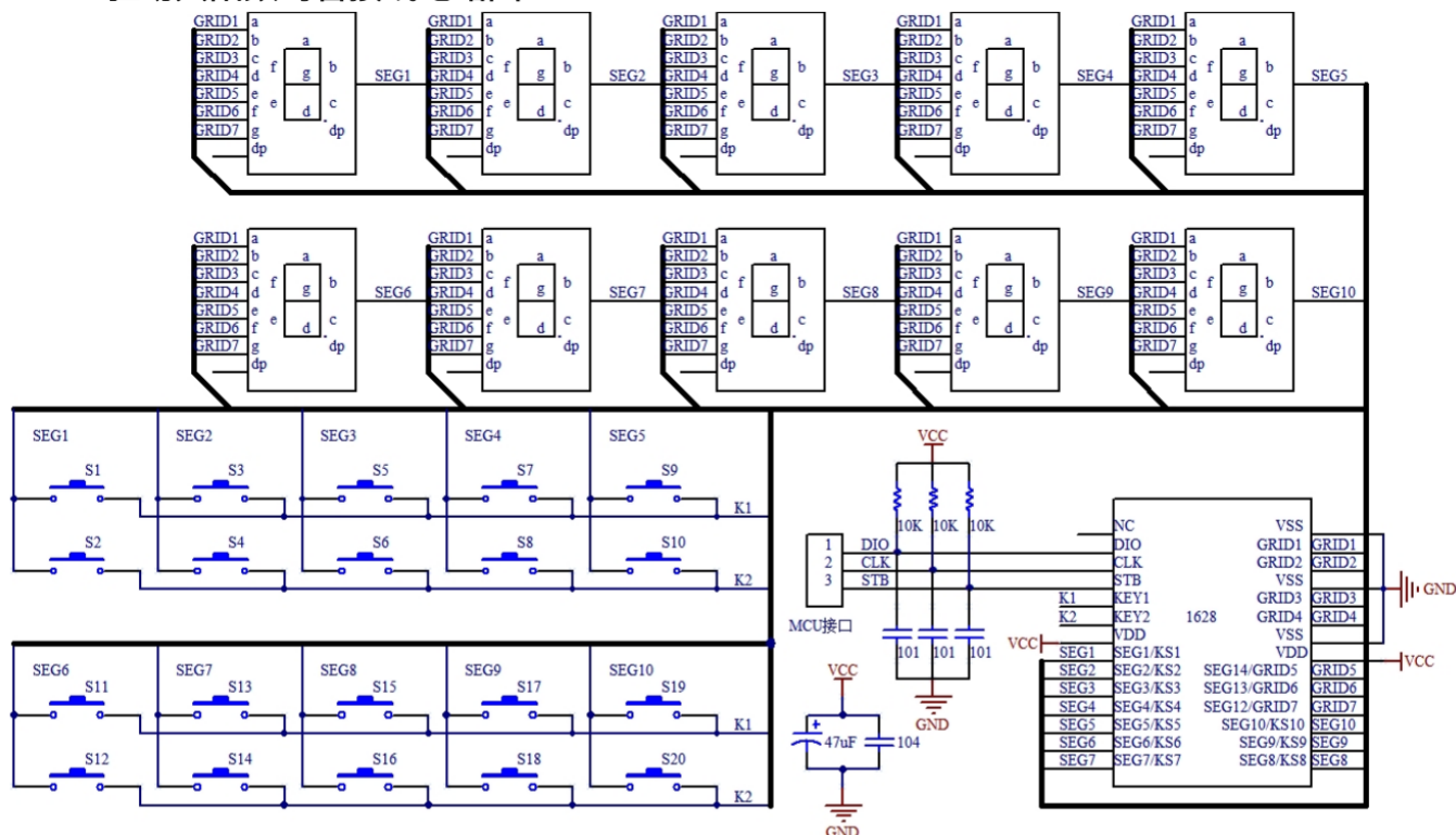
1628驱动共阳数码管接线电路图:
