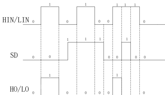
图 8-3. 输入 SD 和输出信号逻辑功能图
