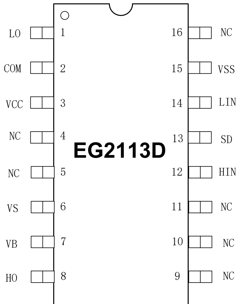
图 4-1. EG2113D 管脚定义
