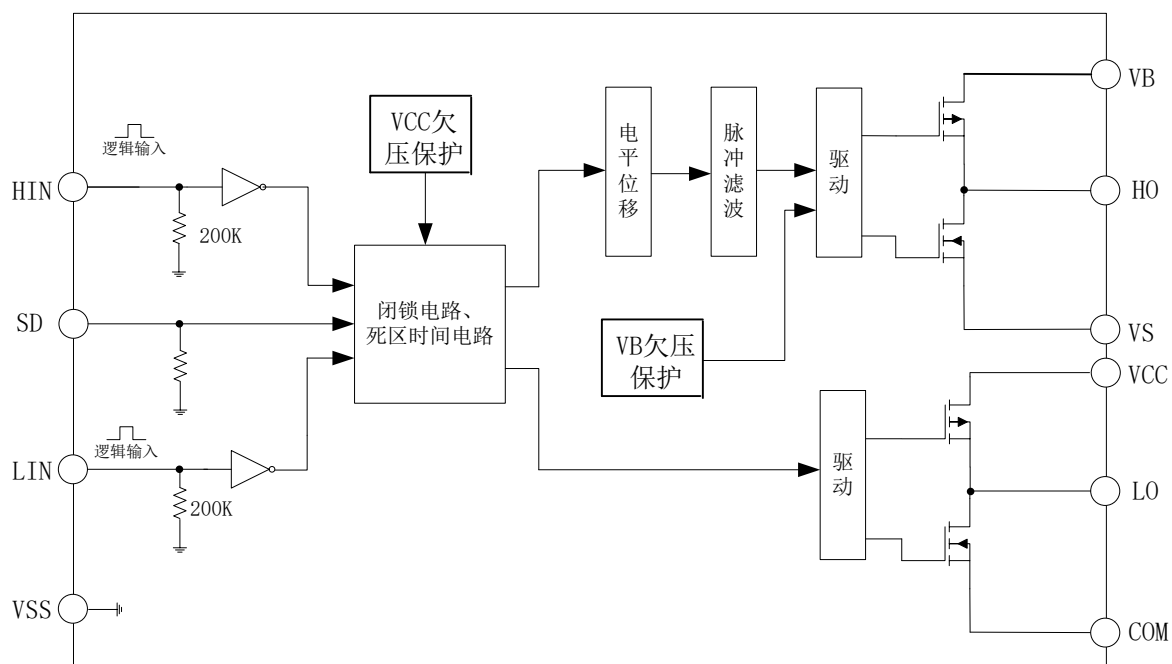
图 5-1. EG2113D 内部电路图
