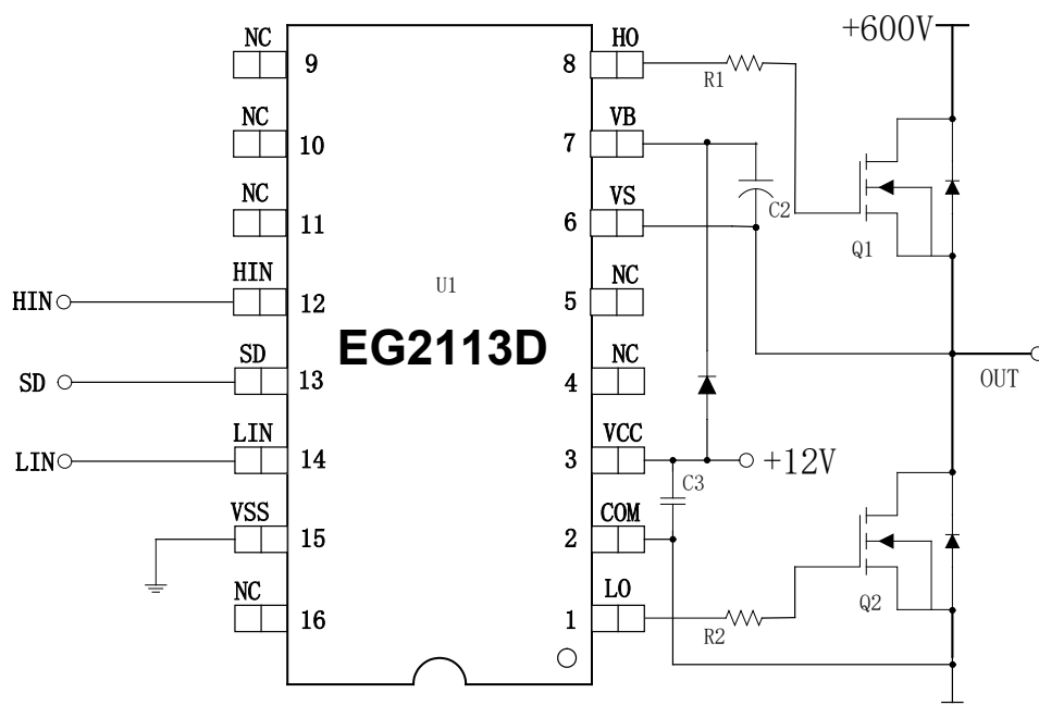
图 6-1. EG2113D 典型应用电路图
