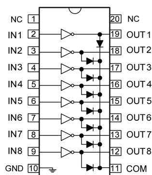
TSSOP-20
