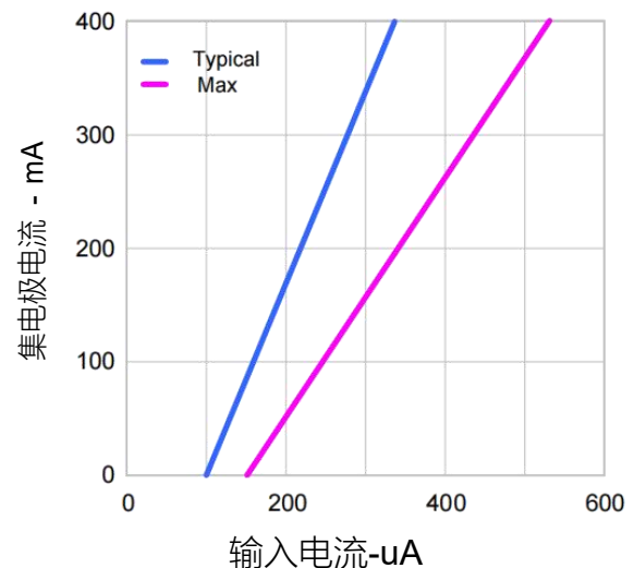
图 2、集电极电流 vs.输入电流
