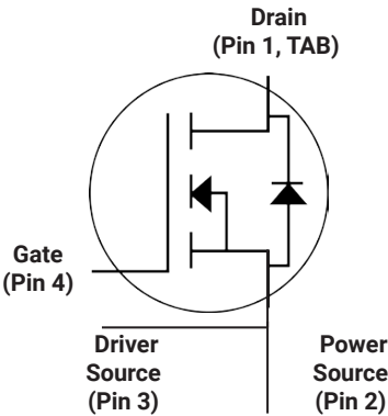
TO-247-4 Package
