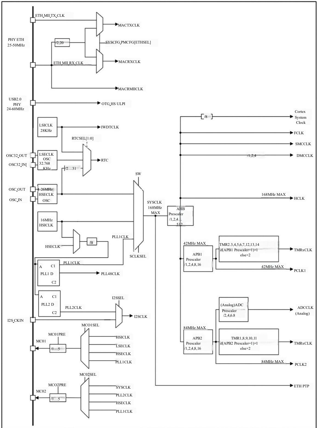
图 7 TD32F407VGT6-TD时钟树
