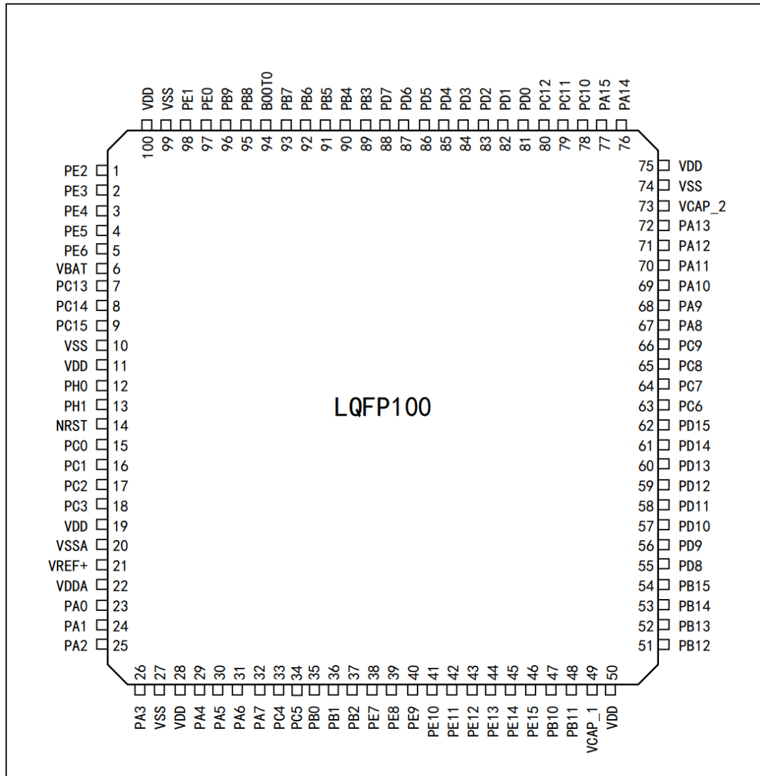
图 3 TD32F407VGT6-TD系列LQFP100 引脚分布图
