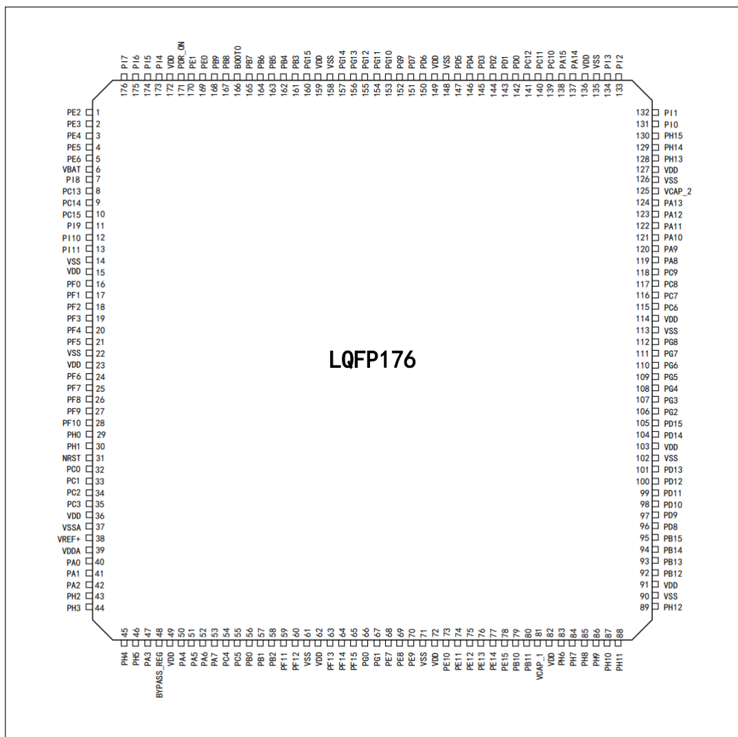
图 1 TD32F407VGT6-TD系列 LQFP176引脚分布图
