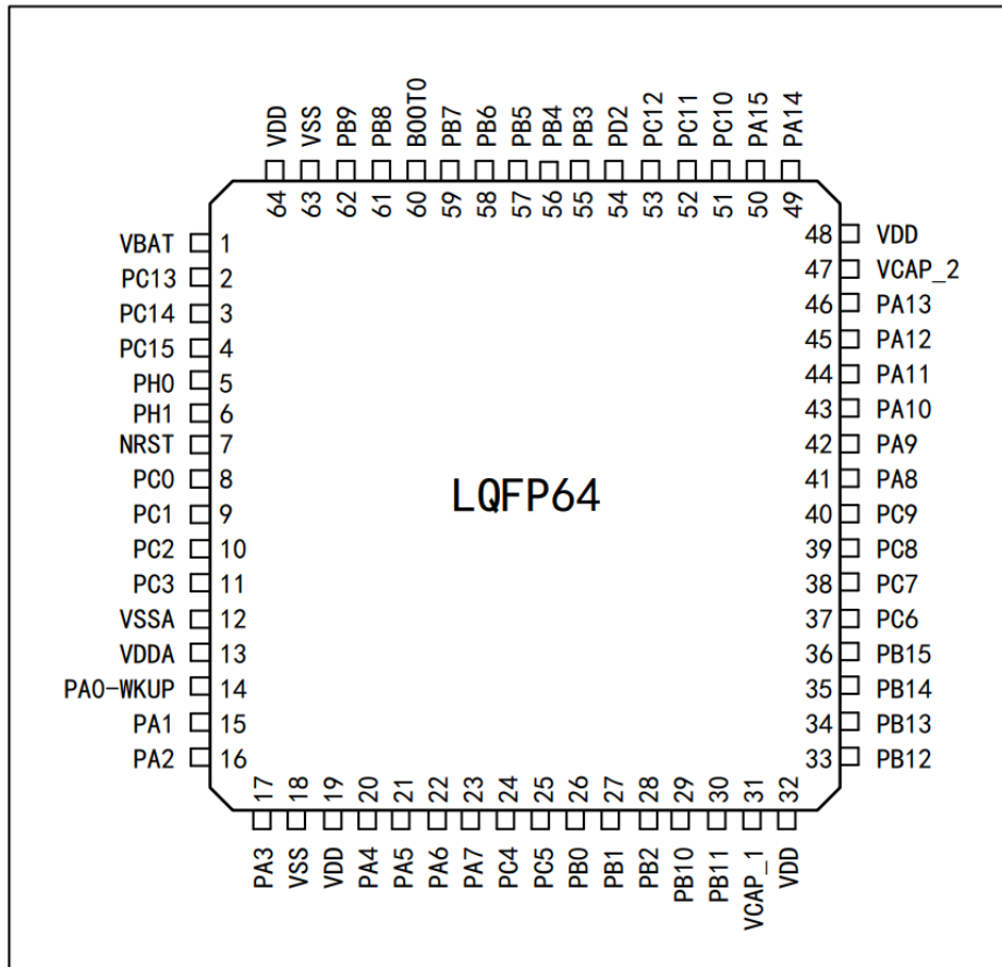
图 4 TD32F407VGT6-TD系列 LQFP64引脚分布图
