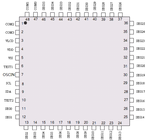
LQFP48
