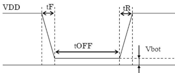
图 2 上升波形图
