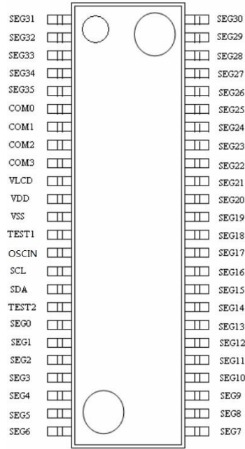
TSSOP48 / SSOP48
