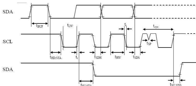
图1 双线通讯交流参数图
