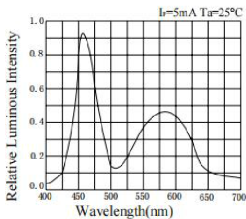
e) 相对光强—波长 e) RELATIVE INTENSITY VS. WAVELENGTH
