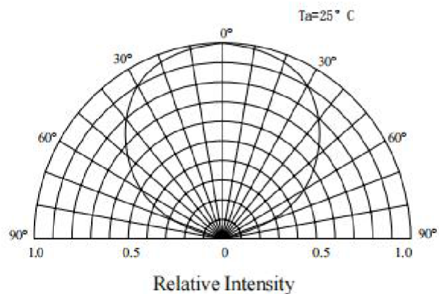
f) 辐射图 f) RADIATION PATTERN
