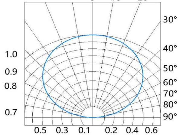
相对辐射强度与空间角度关系 Radiation diagram
