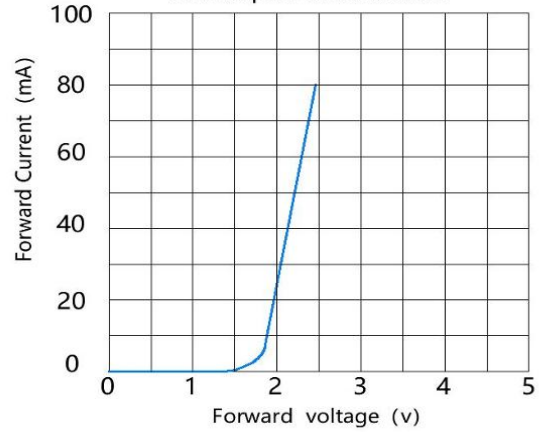
伏安特性 Volt ampere characteristic
