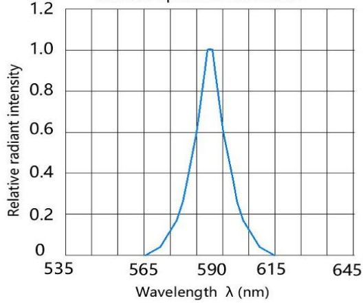
光谱分布曲线 Relative Spectral Distribution
