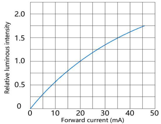
相对光强与正向电流特性 Relative Luminous VS Forward Current
