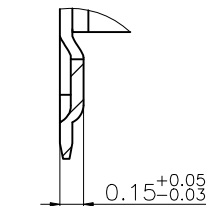
DETAIL:C SCALE 2:1
