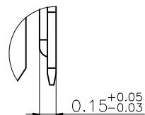
DETAIL:B SCALE 2:1
