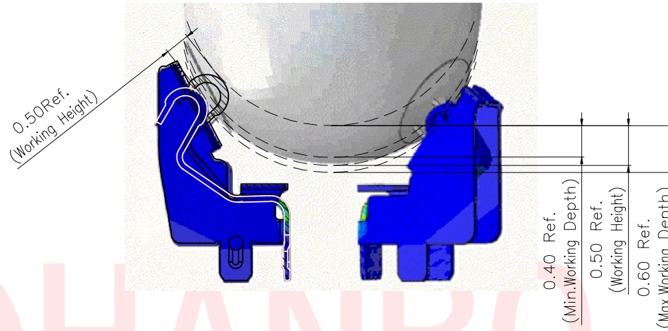
耳机插入示意图(仅供参考)
