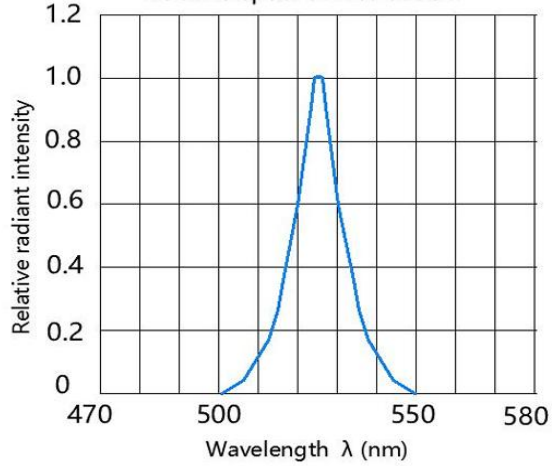
光谱分布曲线 Relative Spectral Distribution
