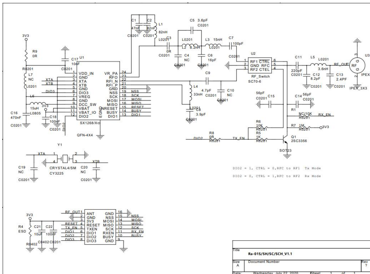
图 6 原理图
