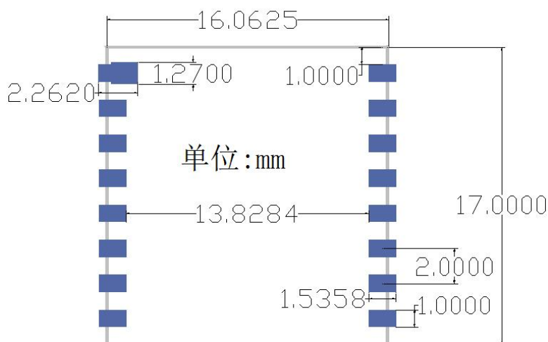
图 9 推荐 PCB 封装尺寸图
