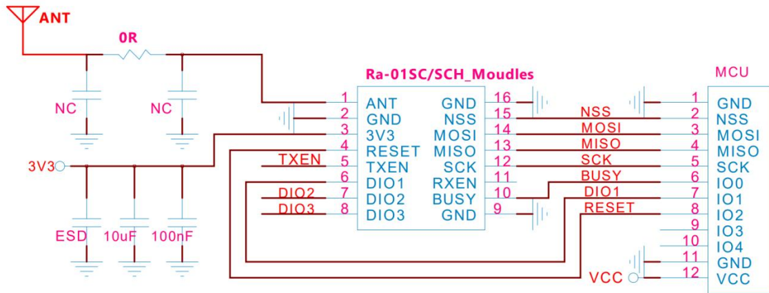
图 7 应用指导电路
