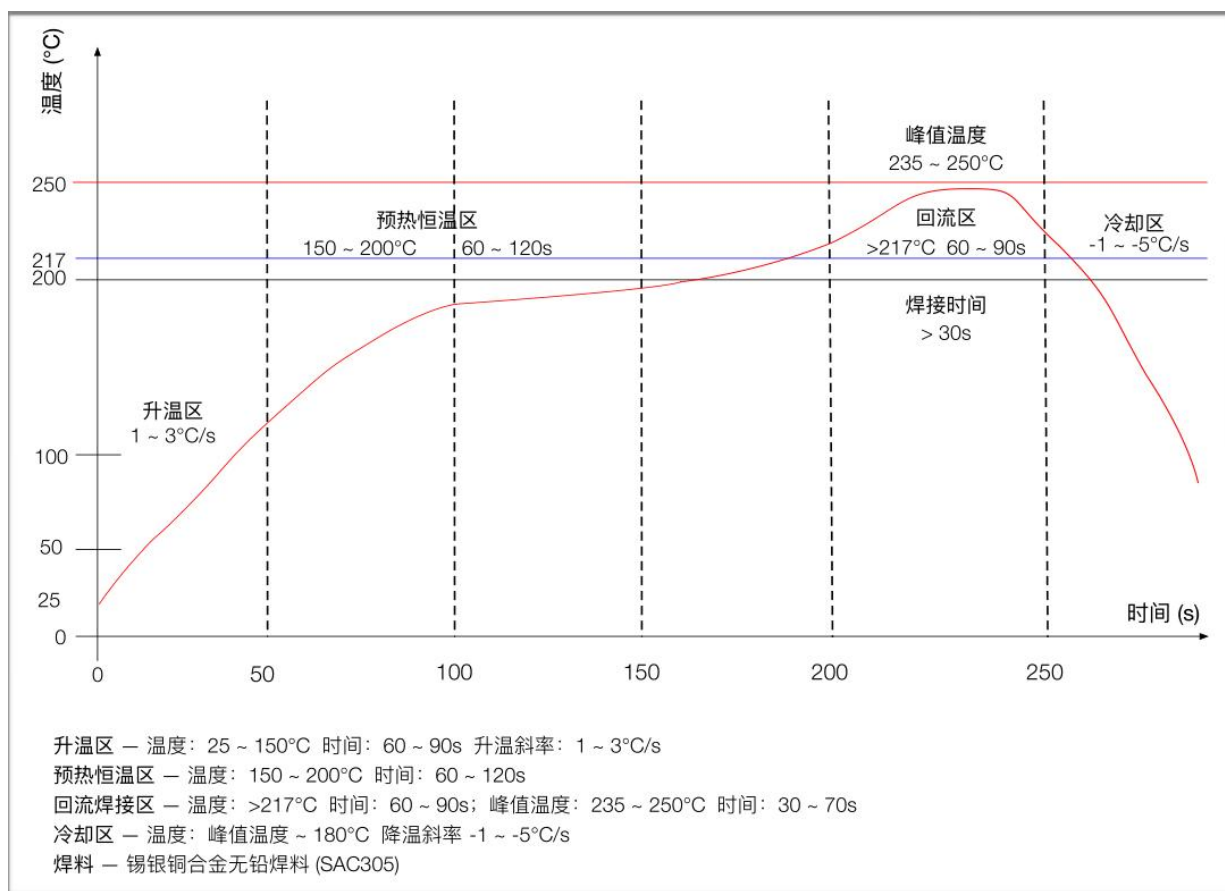
图 12 回流焊曲线
