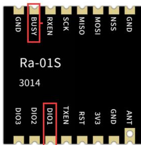
图 8 BUSY/DIO1 应用注意事项
