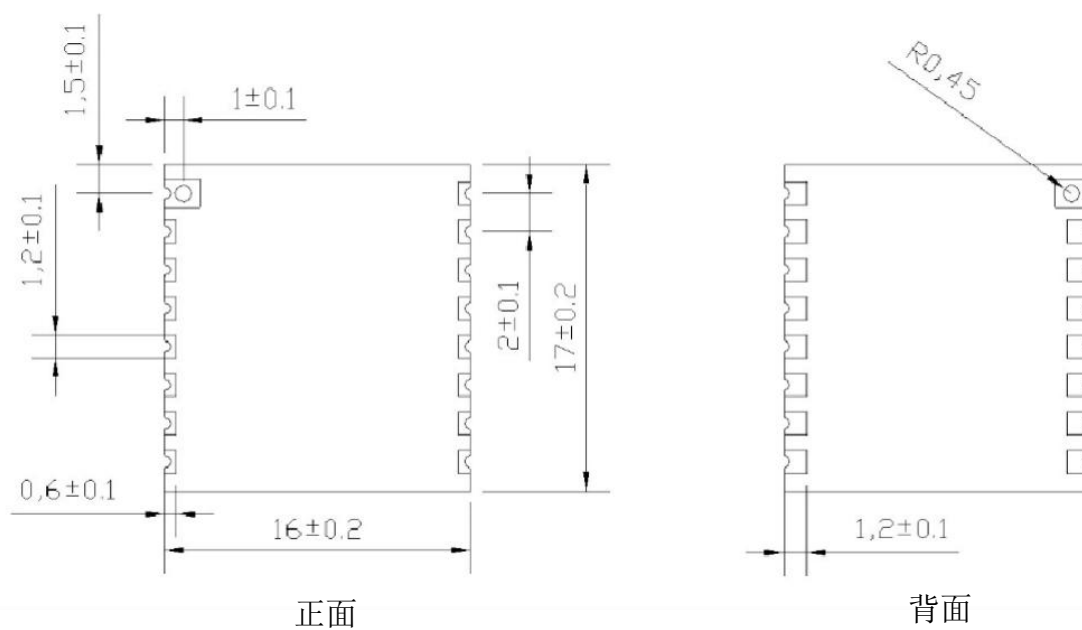
图4 尺寸图
