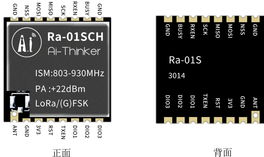
图 5 管脚示意图
