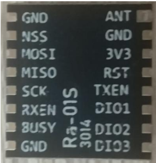
图4 Ra-01S（SX1262 IPEX）管脚示意图
