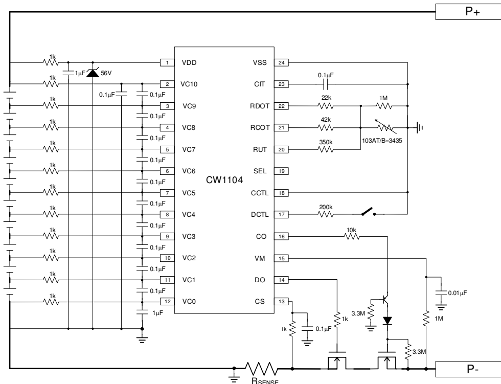
10 串同口应用电路 (电子锁)
