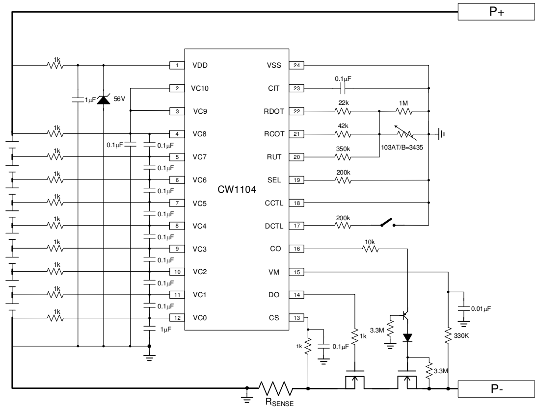
8 串同口应用电路（电子锁）
