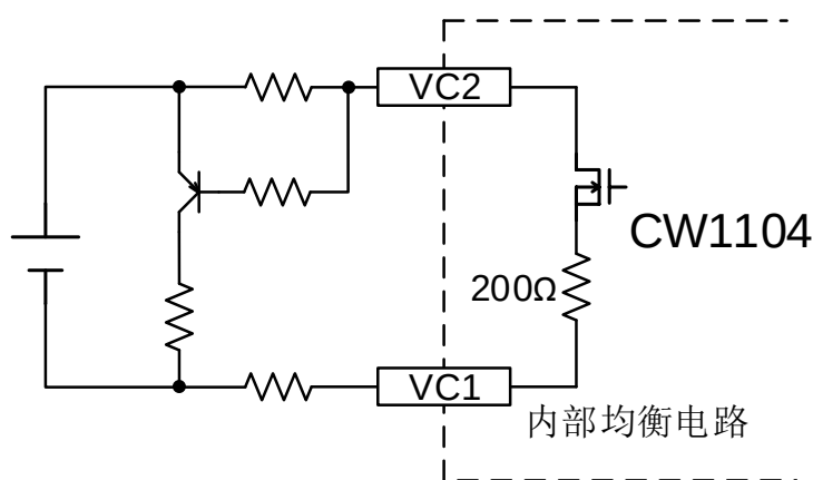
均衡功能示意图
