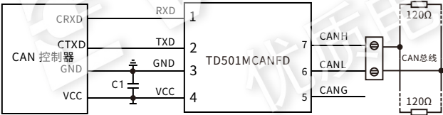
图 1.CAN控制器 5V供电应用电路
