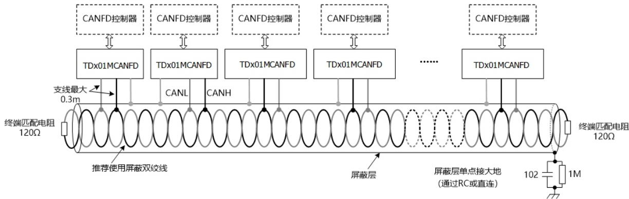
图3.单个CANFD-Bus典型网络连接示意图
