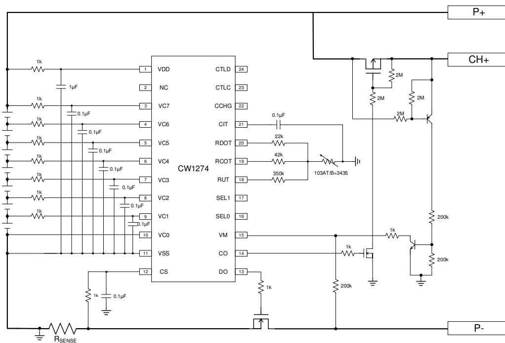
7 串异口应用电路 (CH+)
