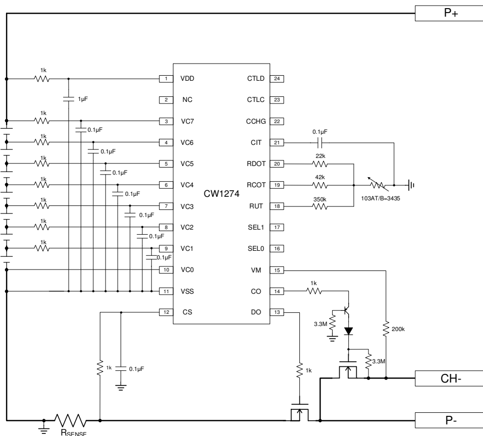
7 串异口应用电路 (CH-)
