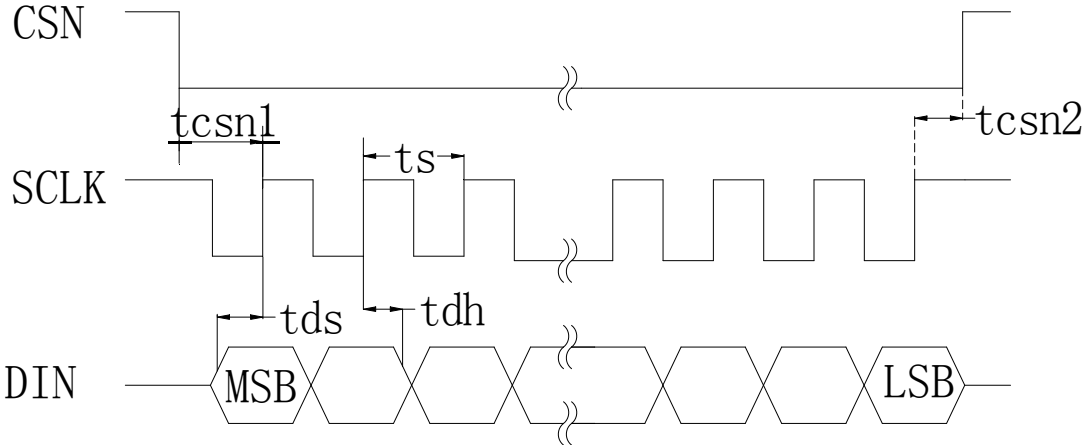
图 3写时序
