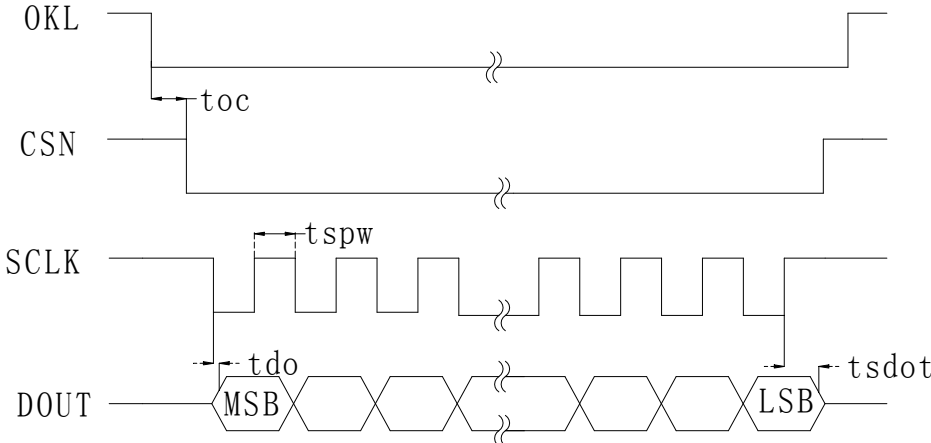
图4读时序
