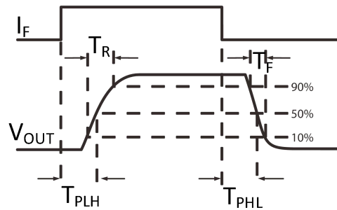
Figure.18 T_{PHL} 、 T_{PLH} 、 T_R 、 T_F Test Circuit
