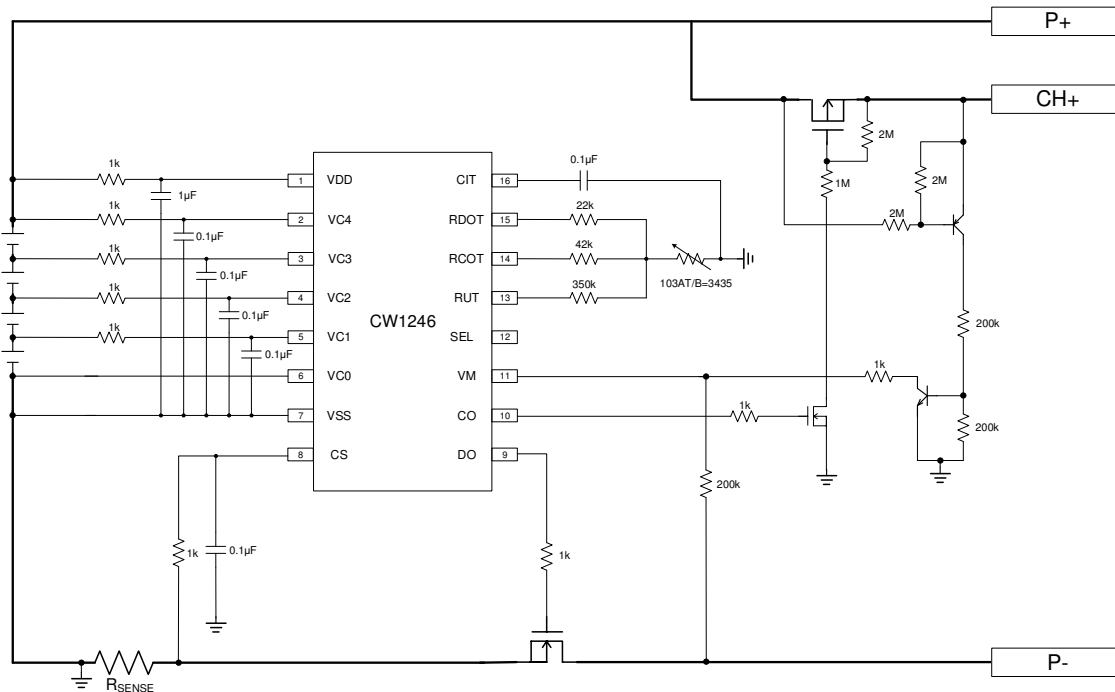
4 串异口应用电路 (CH+)
