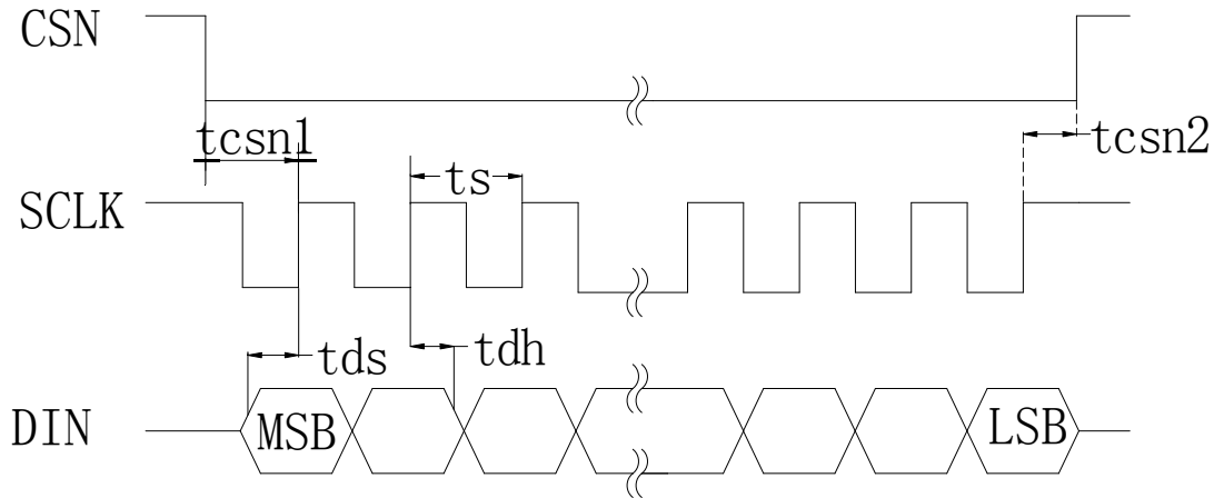
图 3写时序
