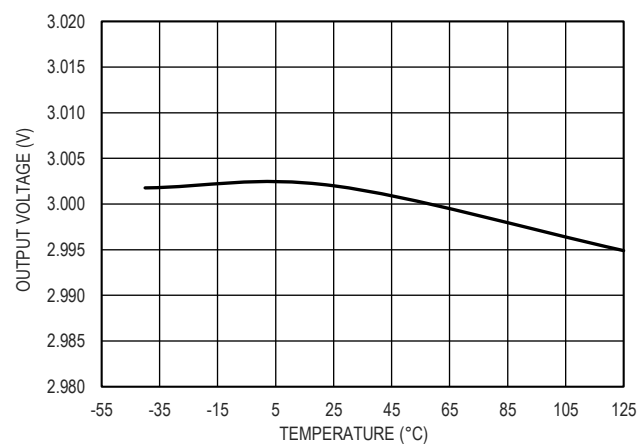
图 12. 3.0V 输出电压精度
