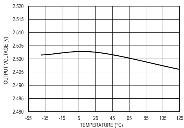
图 11. 2.5V 输出电压精度
