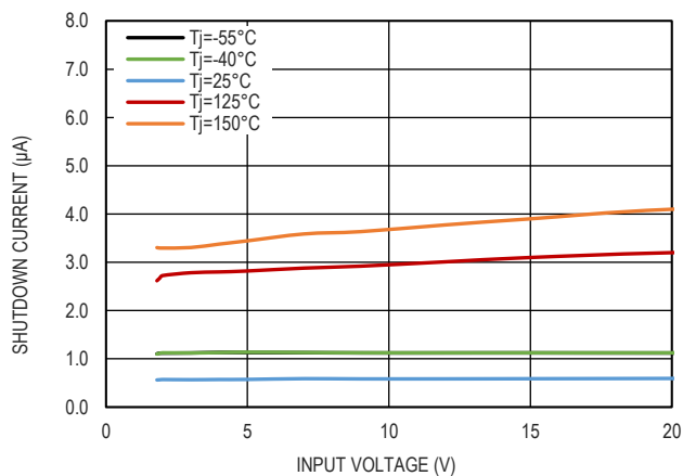
图 4. 关机电流和输入电压的关系
