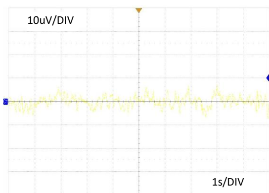
图 17. 1.2V 输出 0.1-Hz to 10-Hz 噪声
