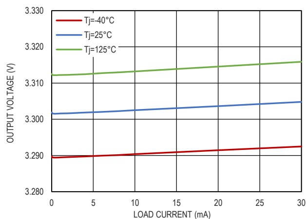
图 9. 3.3V 输出电压和负载电流的关系
