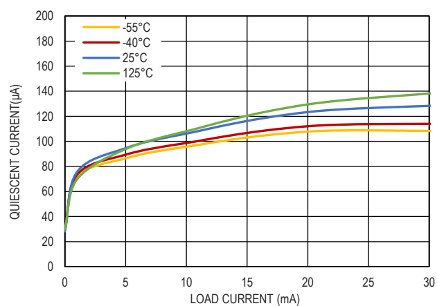
图 5. 静态电流和负载电流的关系, V_{IN} = 4.3V
