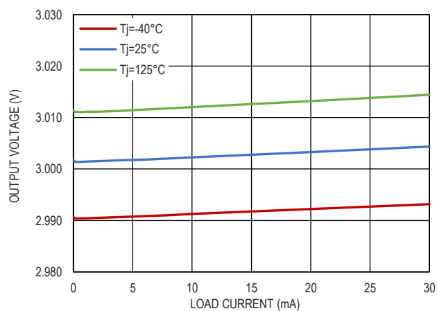
图 8. 3.0V 输出电压和负载电流的关系
