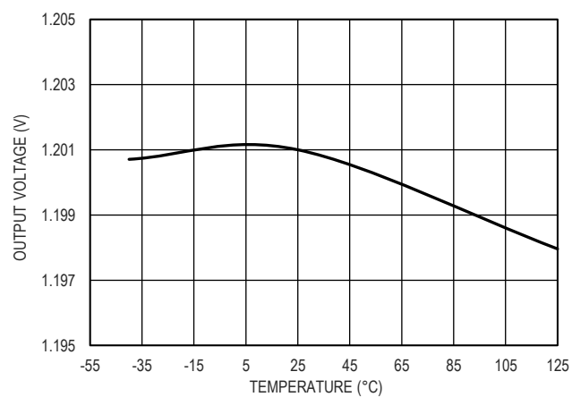
图 10. 1.2V 输出电压精度
