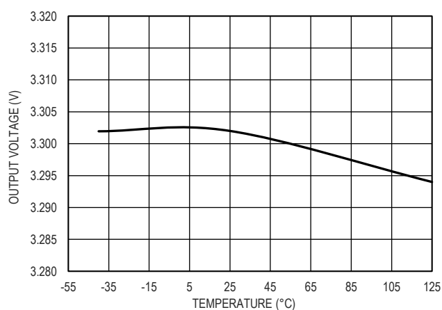
图 13. 3.3V 输出电压精度
