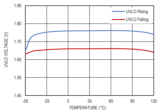
图 14. UVLO 阈值和温度的关系
