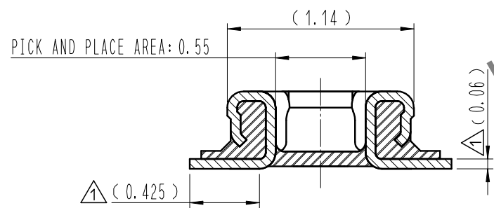
A-A (30:1)
